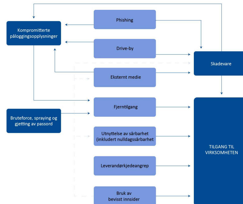
Figur 2: Angrepsvektorer for initiell tilgang [5], [6].
